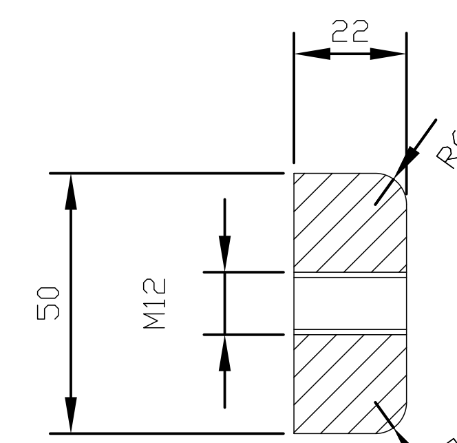
Sez. 2-2
