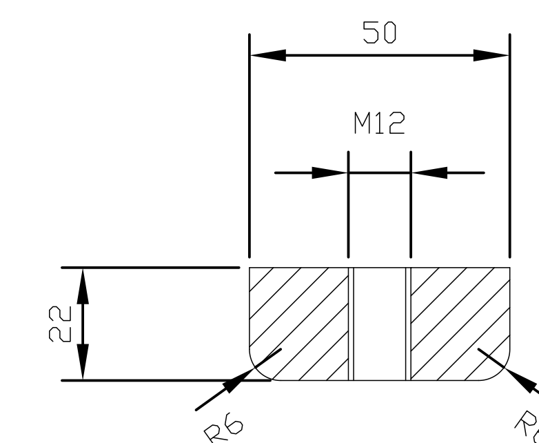
Sez. 1-1
