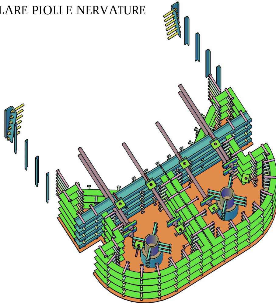
PARTICOLARE PIOLI E NERVATURE
