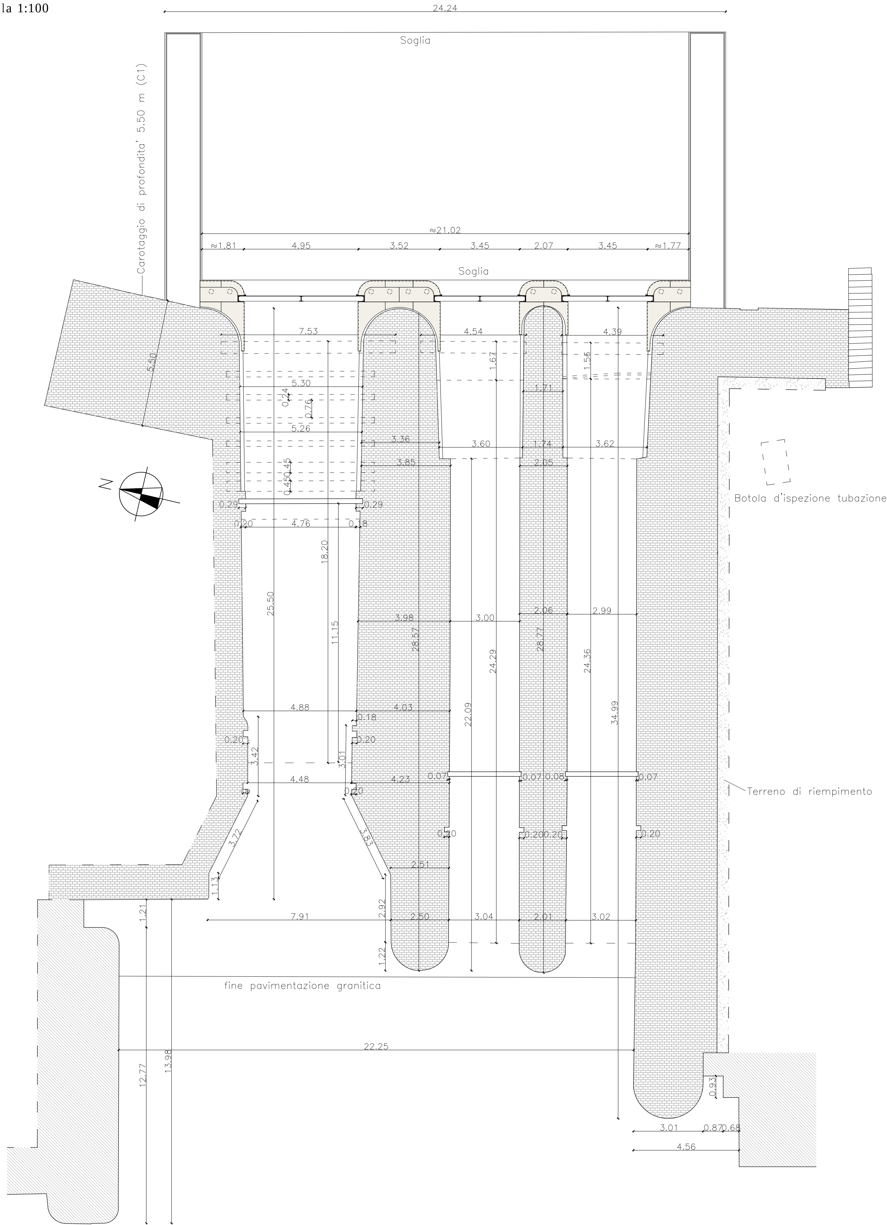
PIANTA Scala 1:100
