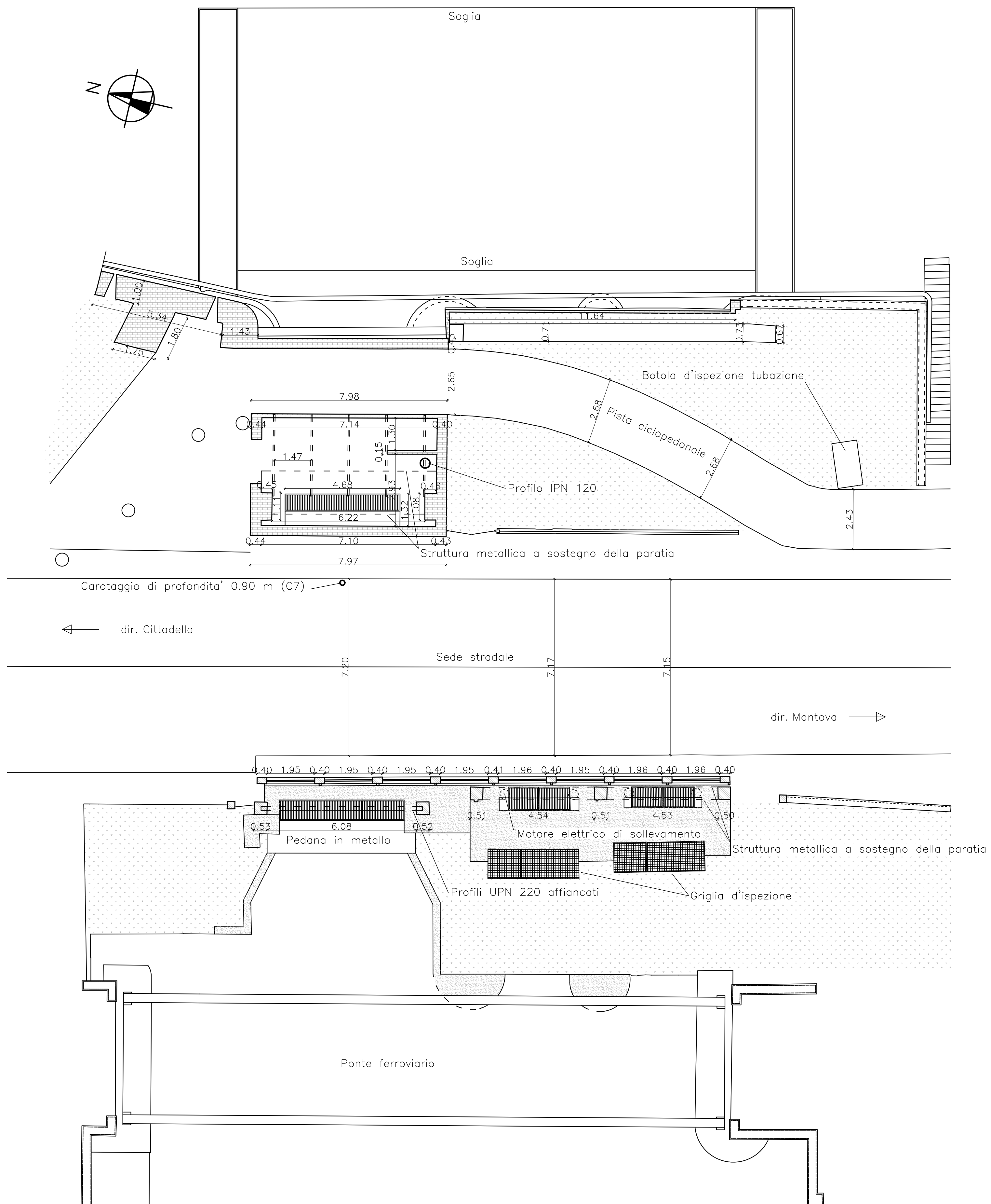
INDIVIDUAZIONE IN PLANIMETRIA DELLA PIANTE COPERTURA P3 SCALA 1:200
