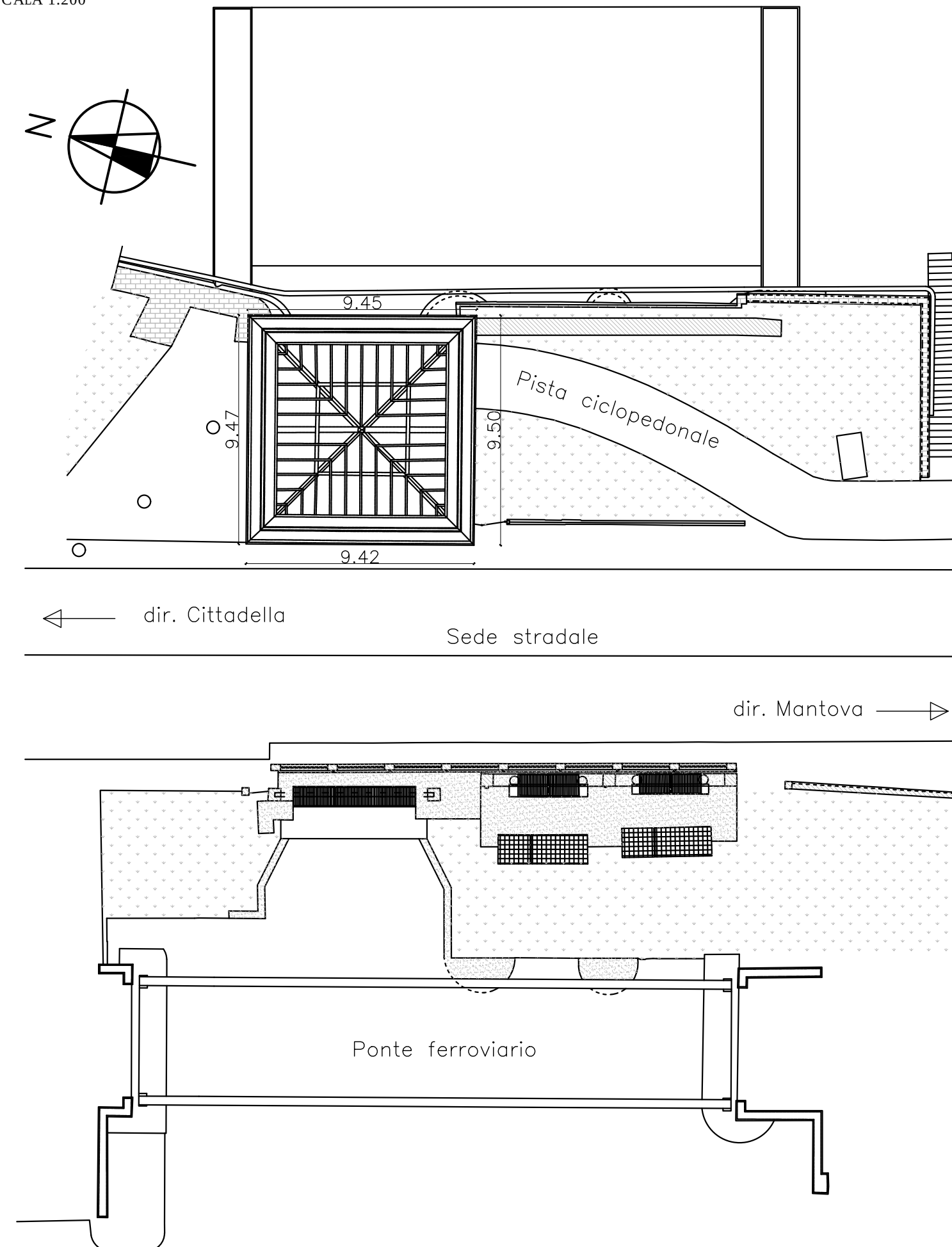
INDIVIDUAZIONE IN PLANIMETRIA DELLA PIANTE COPERTURA P3 SCALA 1:200
