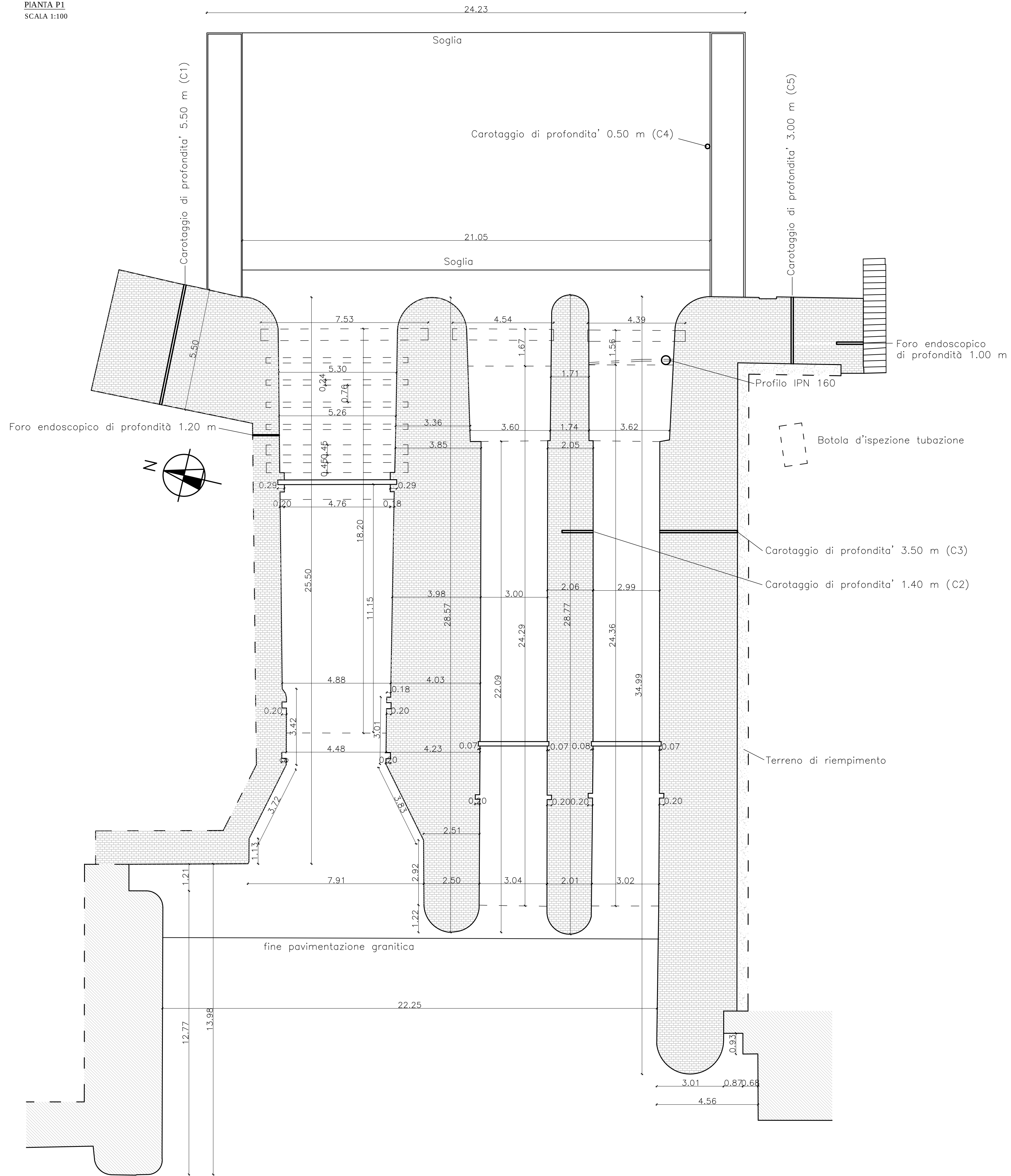
PIANTA P1 SCALA 1:100
