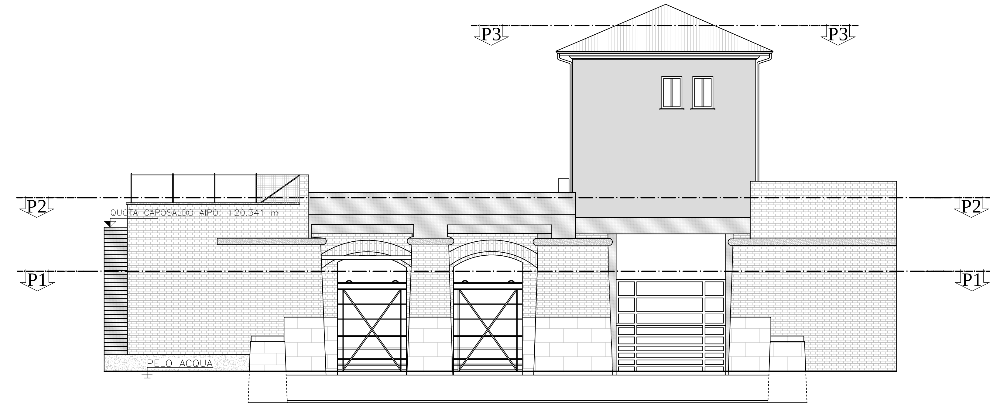
PROSPETTO LATO VALLE CON INDICAZIONE DELLE PIANTE SCALA 1:100
