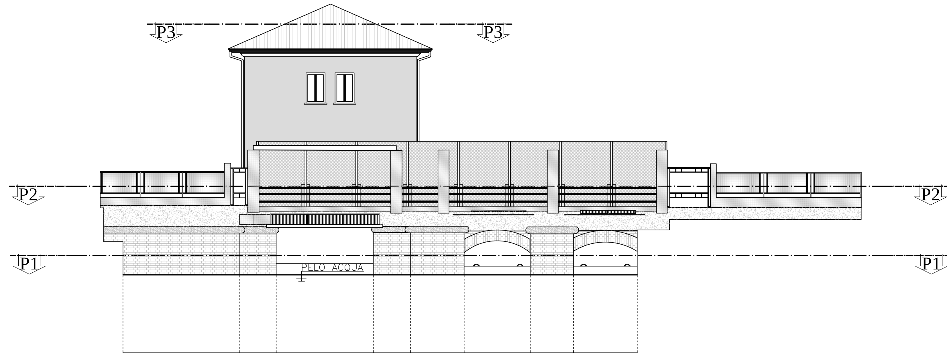
PROSPETTO LATO MONTE CON INDICAZIONE DELLE PIANTE SCALA 1:100
