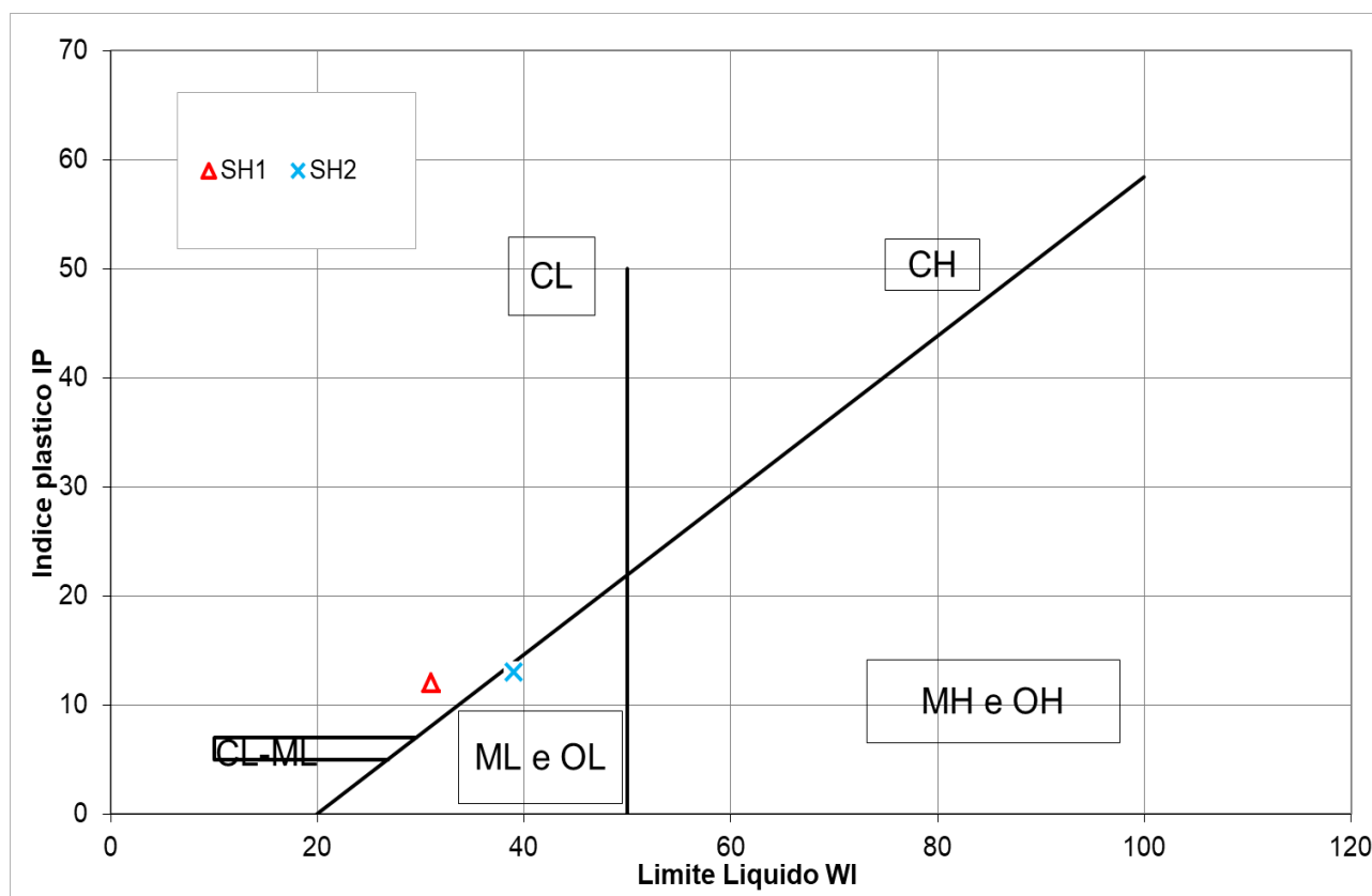
Fig. 8 – Carta della plasticità
