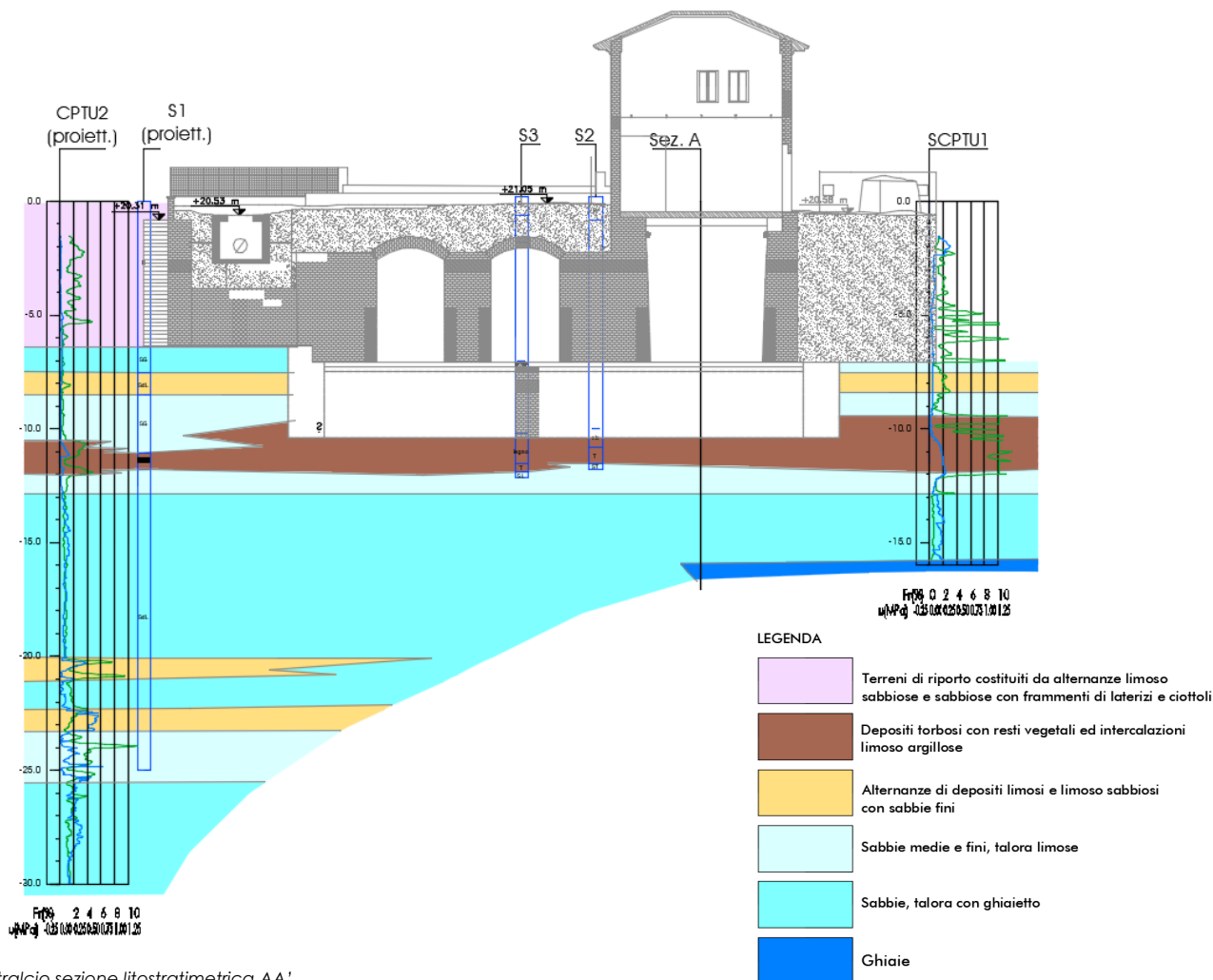
Fig. 18 – Stralcio sezione litostratimetrica AA'
