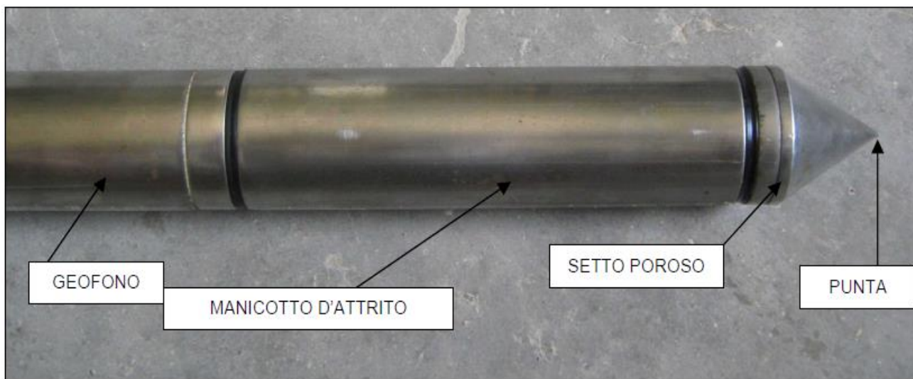
Fig. 12 – Punta del penetrometro elettrico e sismocono
