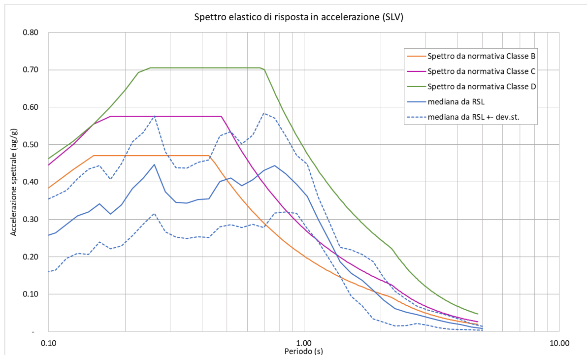
Fig. 37 - Valori mediاني dello spettro elastico di risposta in accelerazione (SLV) confrontato con gli spettri semplificati di normativa (Classi B, C e D)
