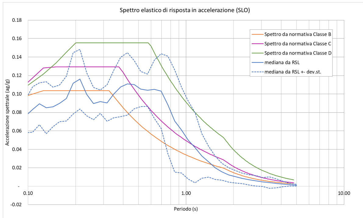
Fig. 39 - Valori mediani dello spettro elastico di risposta in accelerazione (SLO) confrontato con gli spettri semplificati di normativa (Classi B, C e D)
