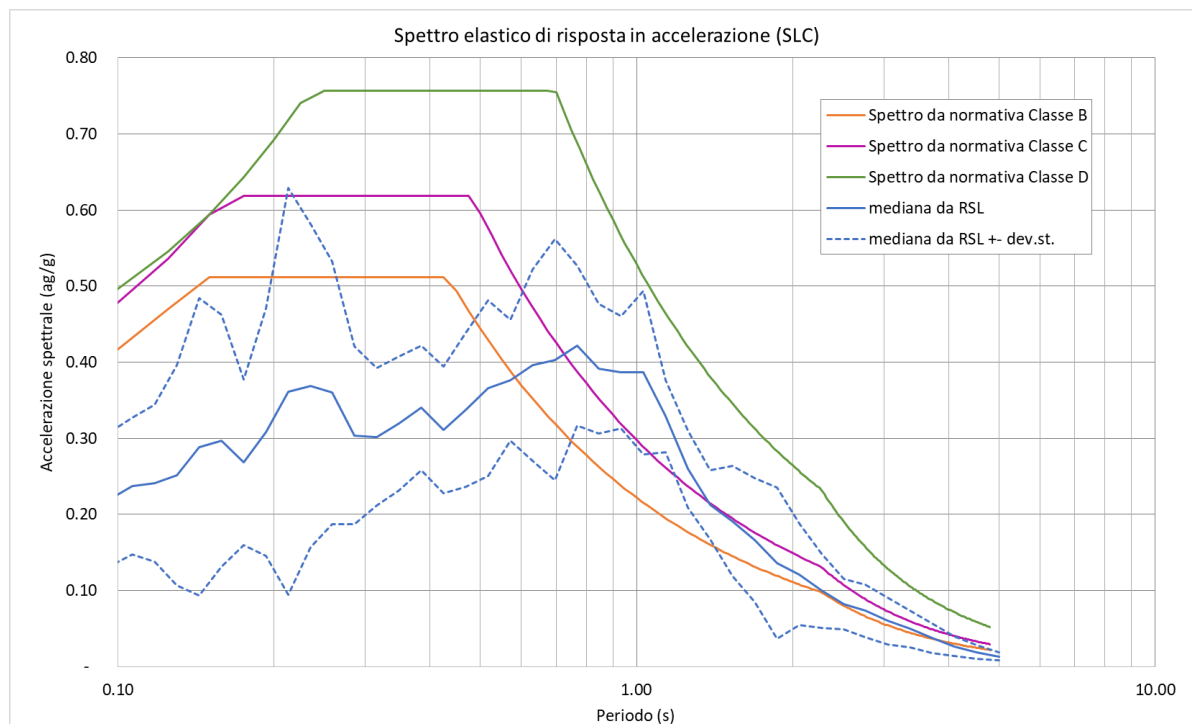
Fig. 38 - Valori mediani dello spettro elastico di risposta in accelerazione (SLC) confrontato con gli spettri semplificati di normativa (Classi B, C e D)
