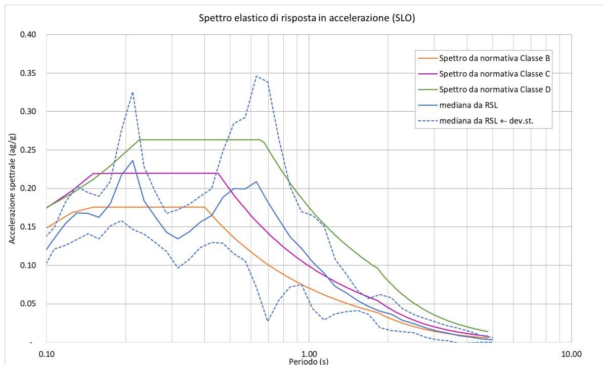
Fig. 36 - Valori mediاني dello spettro elastico di risposta in accelerazione (SLO) confrontato con gli spettri semplificati di normativa (Classi B, C e D)
