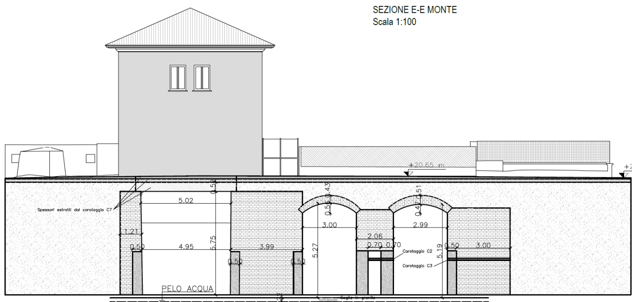
Figura 2-1 – Prospetto da monte delle luci dei canali di scarico
