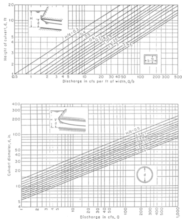
Figura 5-2 - Cartogrammi per la stima delle portate defluibili a pelo libero attraverso tombini scatolari o circolari con imbocco non raccordato
