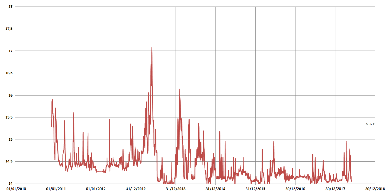
Figura 4-9 -- Livelli idrometrici del lago di Mezzo all'idrometro di Vasarone nel periodo 2010 – 2018
