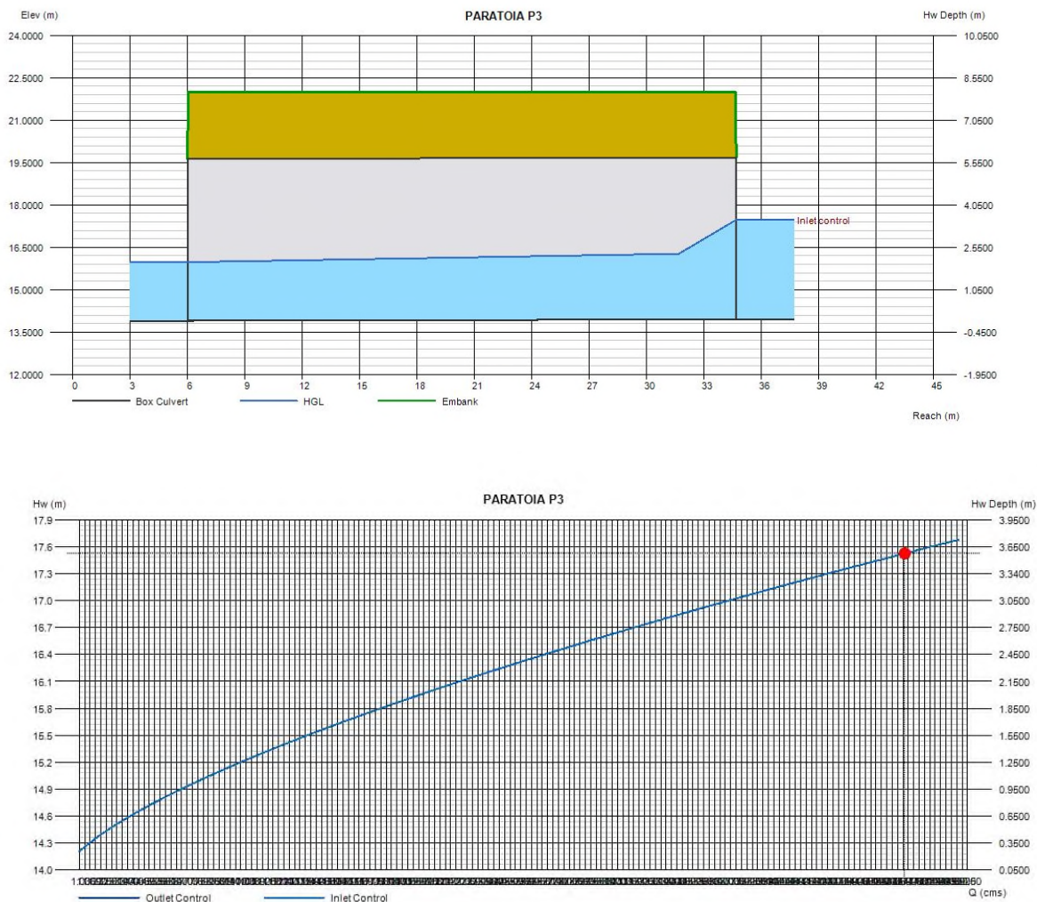
Figura 5-5 – Profilo idraulico e scala di deflusso del canale di scarico relativo alla paratoia P3
