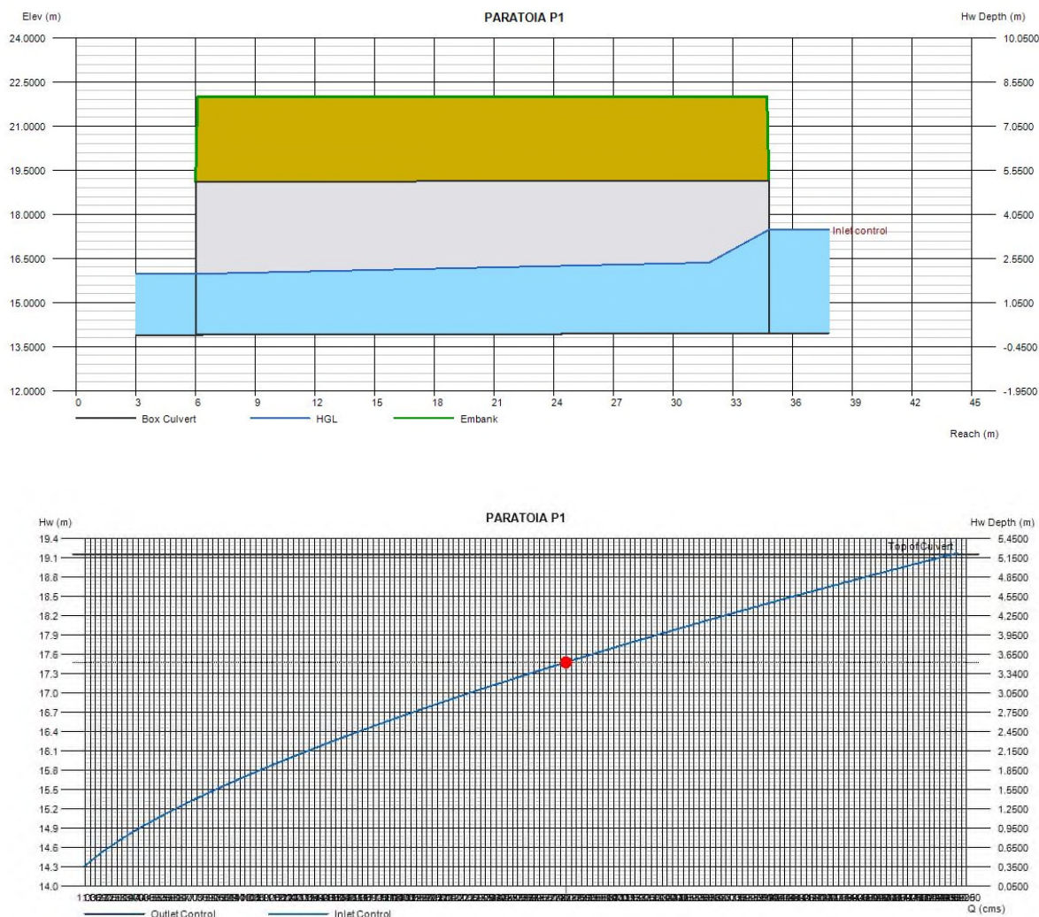
Figura 5-3 – Profilo idraulico e scala di deflusso del canale di scarico relativo alla paratoia P1
