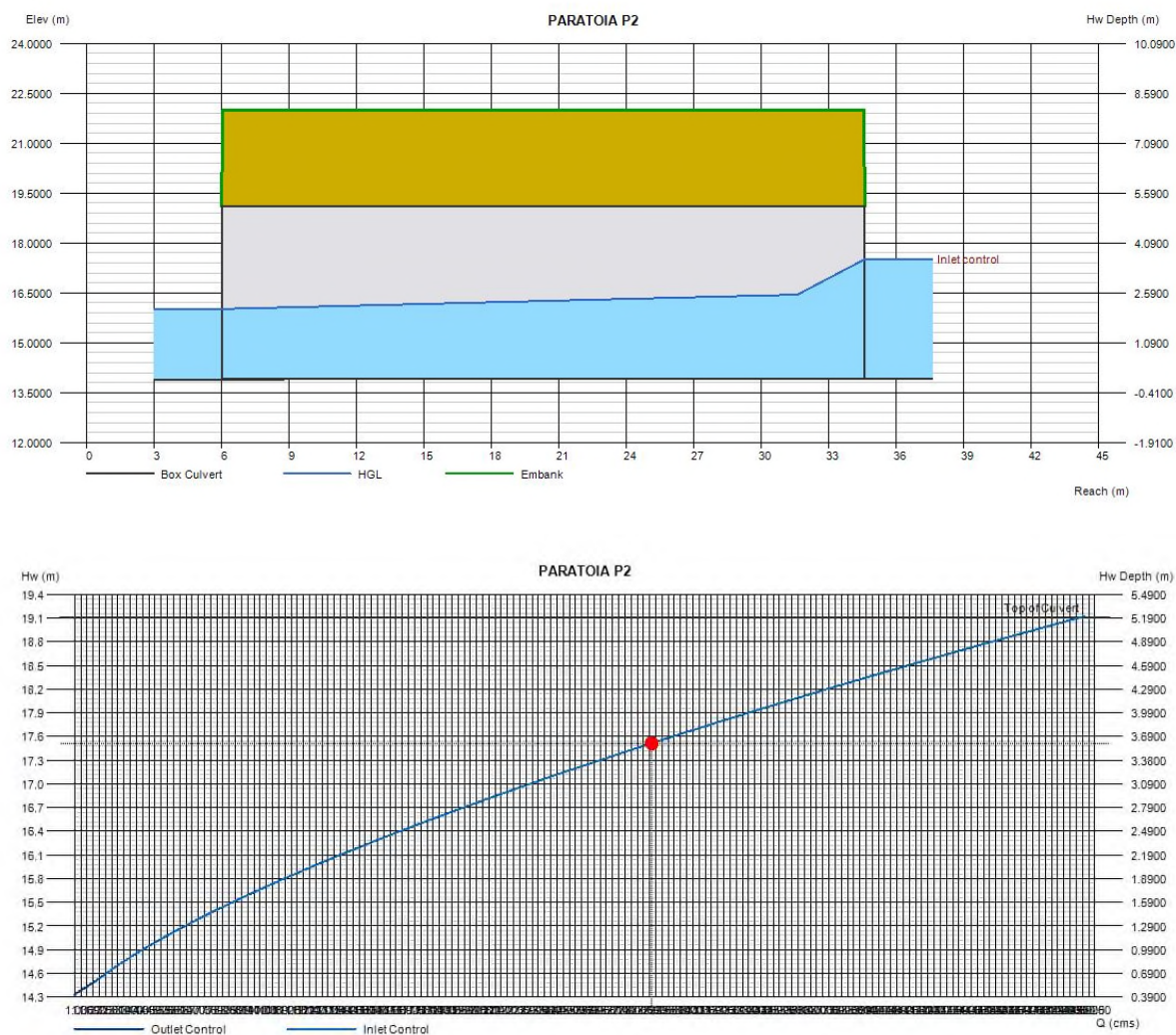
Figura 5-4 – Profilo idraulico e scala di deflusso del canale di scarico relativo alla paratoia P2
