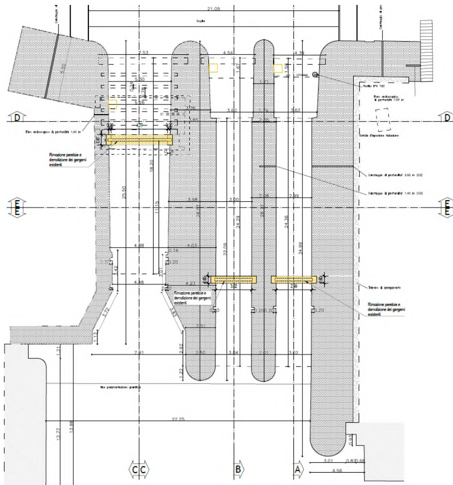
Figura 2-2 – Pianta lungo i canali di scarico del manufatto del Vasarone
