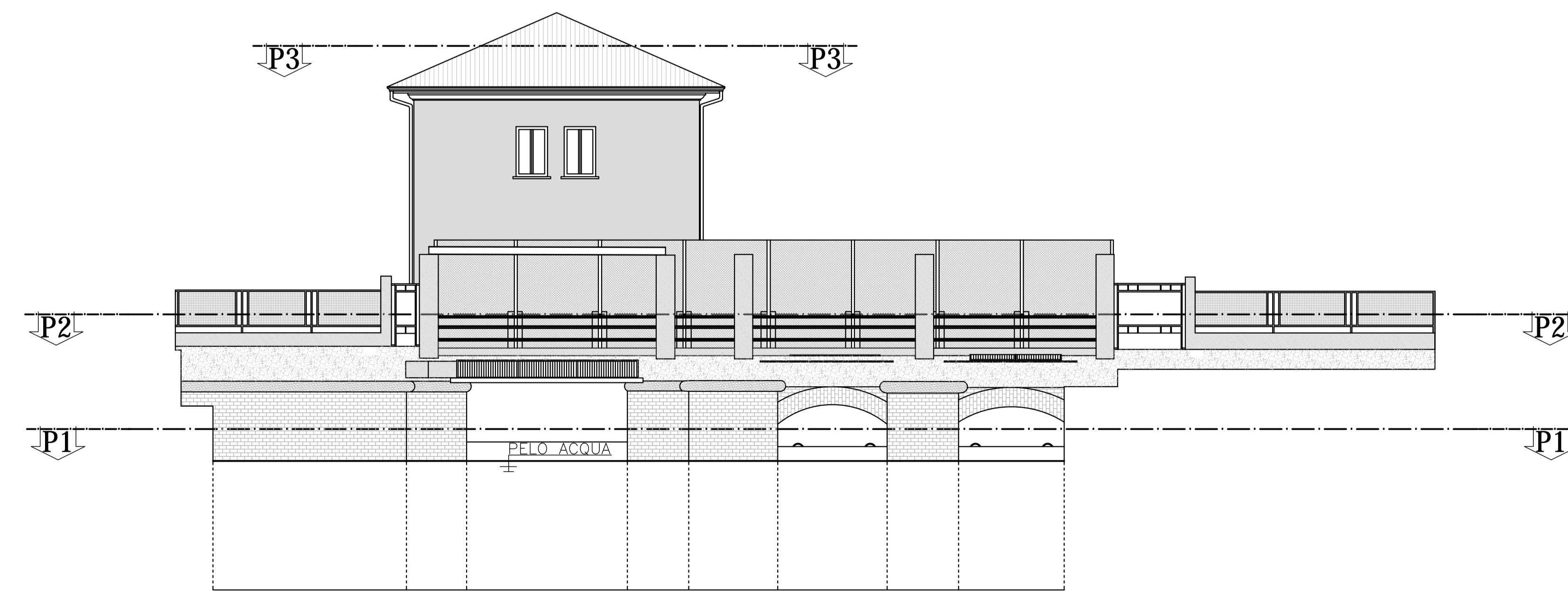
PROSPETTO LATO MONTE CON INDICAZIONE DELLE PIANTE SCALA 1:100
