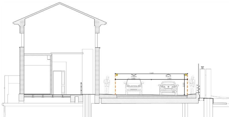
Sezione stradale in corrispondenza dell'edificio di contenimento della paratoia principale – Lotto A
