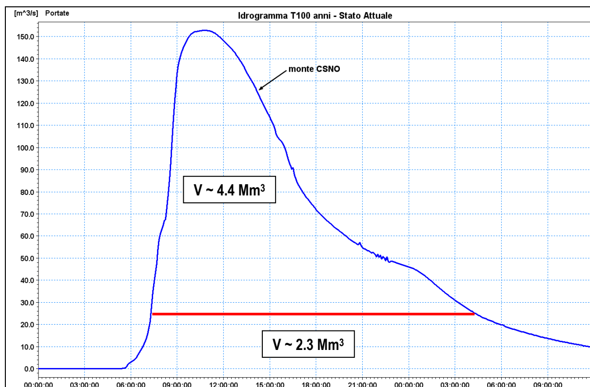
Figura 47 – Idrogramma di piena del T. Seveso a monte della presa del C.S.N.O.. La linea rossa rappresenta il limite della portata che può proseguire nel C.S.N.O. a valle di Senago (intersezione con il T. Garbogera)
