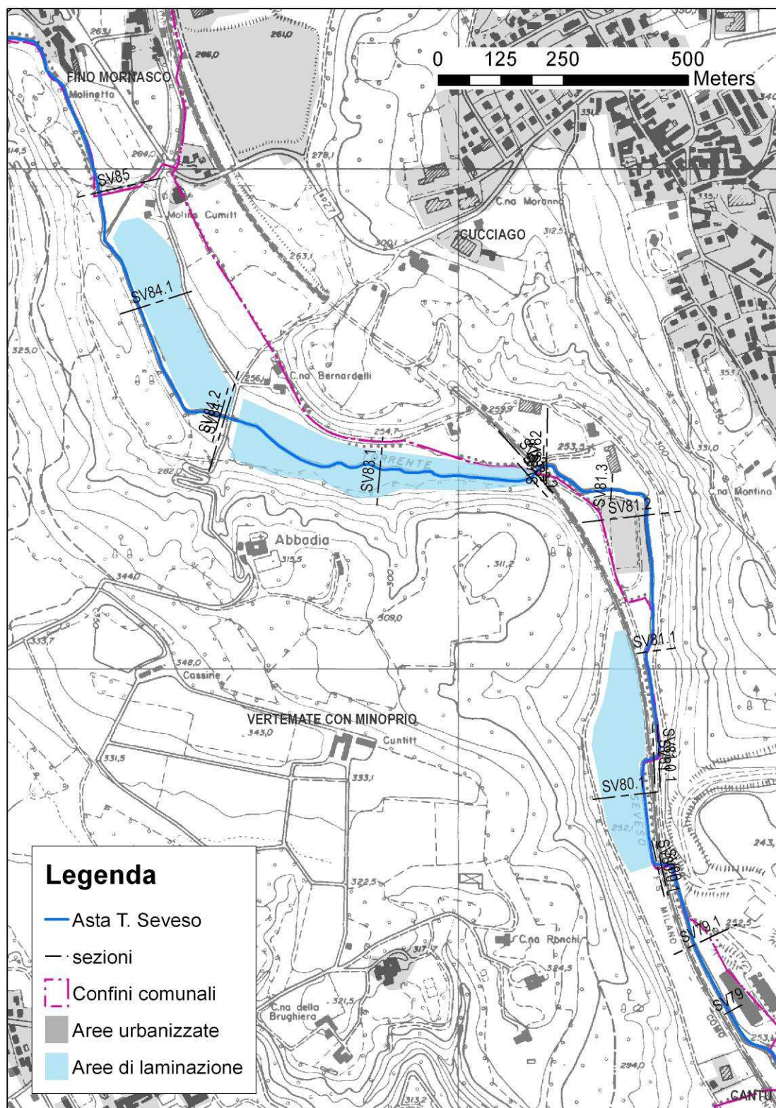
Figura 72 – Aree di laminazione a Vertemate con Minoprio.
