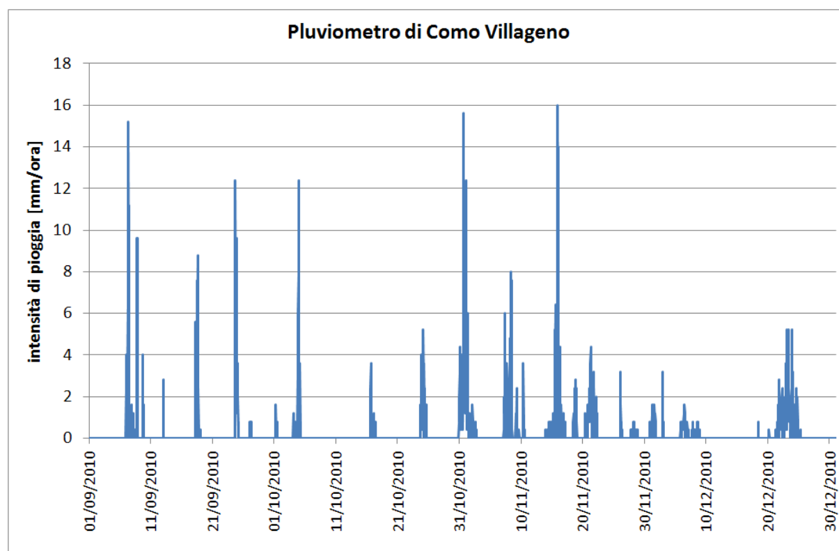
Figura 23 – Dati registrati dal pluviometro di Como Villageno
