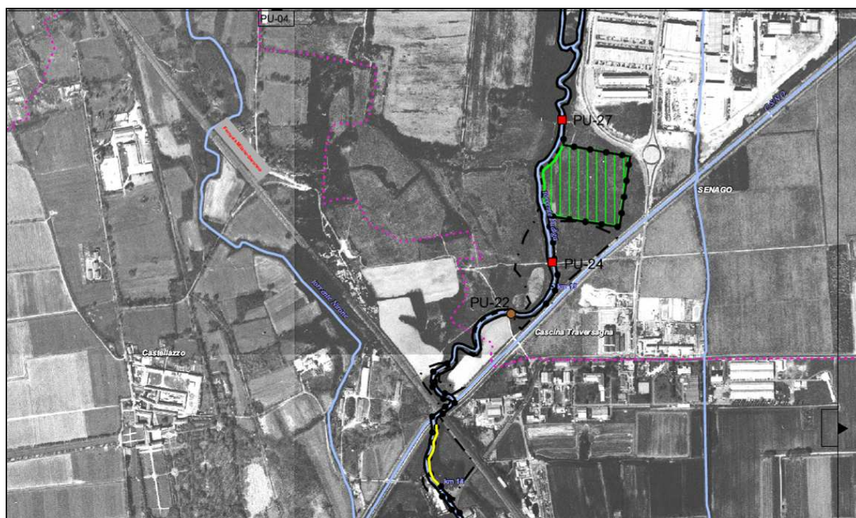
Figura 64 – Stralcio della cartografia degli interventi di sistemazione del T. Pudiga con riportata l'area di laminazione prevista, caratterizzata da una volumetria di 100'000 \text{ m}^3 (AdBPo – 2004).
