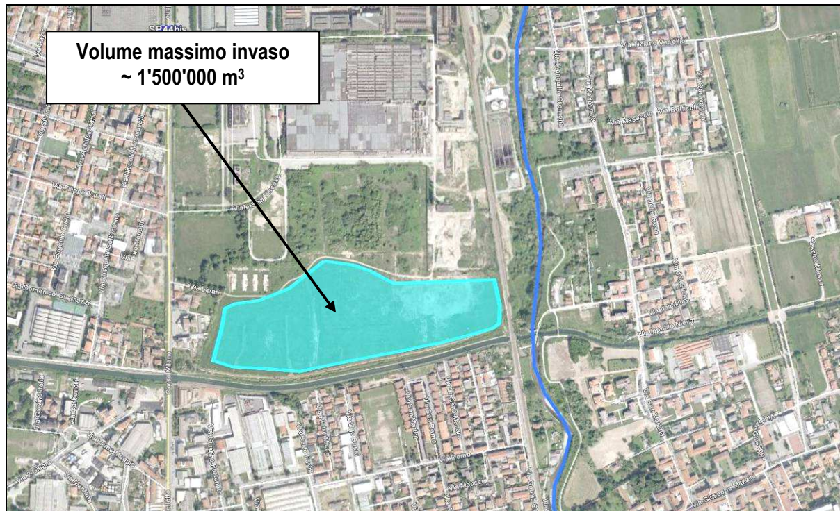
Figura 58 – Invaso di laminazione in comune di Paderno Dugnano, a monte Canale Villoresi
